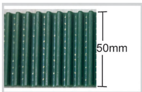
LS/C-360C BANDA PARA BASTIDOR PASO S5M, ANCHO 50MM, # PARTE BPS5M50-®
