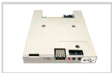
CONVERTIDOR TIPO LAPTOP 720KB, CONEXIÓN MEMBRANA BARUDAN® ,
