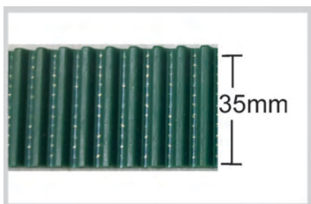
LS/C-360B BANDA PARA BASTIDOR PASO S5M, ANCHO 35MM, # PARTE BPS5M35-® 623500360000®
