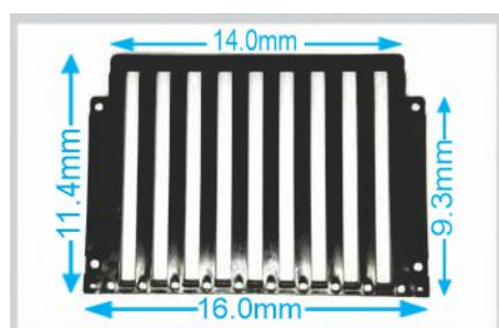
LS-2204 REJILLA PARA 9 COLORES ALTA
