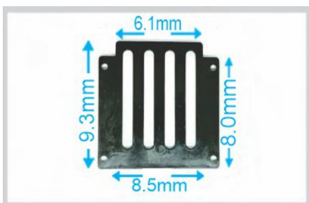
LS/B-096 REJILLA 4 COLORES
