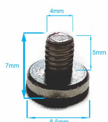
TORNILLO MODELO 308AB, ALTO 7MM, CABEZA 8.5MM, CUERDA 4MM, ALTO CUERDA 5MM
