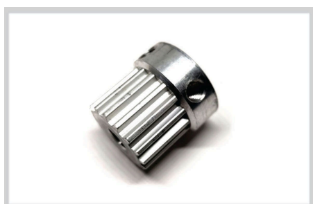
WS282 POLEA PARA NEO® S5M 17MM, Z16, 50143012S10®
