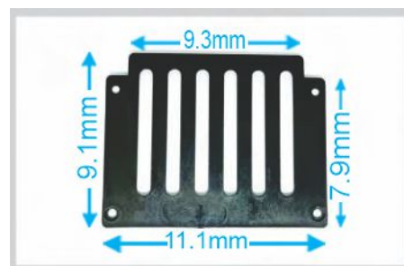
LS/B-097 REJILLA 6 COLORES # PARTE EF0607000600*
