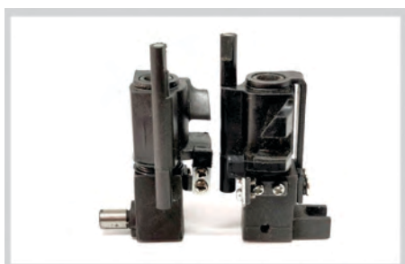
LS/E-021 SET DE CATCHER, PARA MAQ. CHINAS 1 CABEZA CON MOTOR DE SALTA PUNTO
