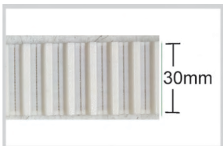
LS/C-360D BANDA PARA BASTIDOR PASO T10, ANCHO 30MM
